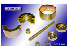
Ściągacz piasty / łożyska VAG z i bez ABS
