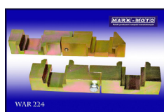
Blokada wałków rozrządu BMW benzyna M60 / M62
