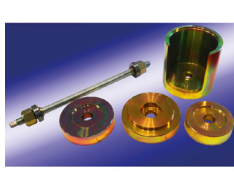
Ściągacz tulei tylnej belki (środkowa) BMW 5 (E60, E61) BMW 6 (E63, E64)
