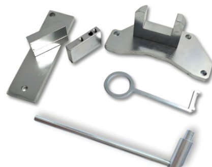
Blokada rozrządu 1,2 VTI (VVT) / GDI po 2018 mokry pasek PSA / Opel / Toyota
