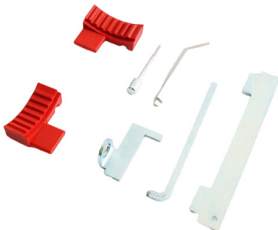
Blokada rozrządu 1,4 / 1,6 / 1,8 16V Twinsport Opel / Fiat / Chevrolet / Alfa Romeo Cena: 99,31 zł Symbol: HST 246
